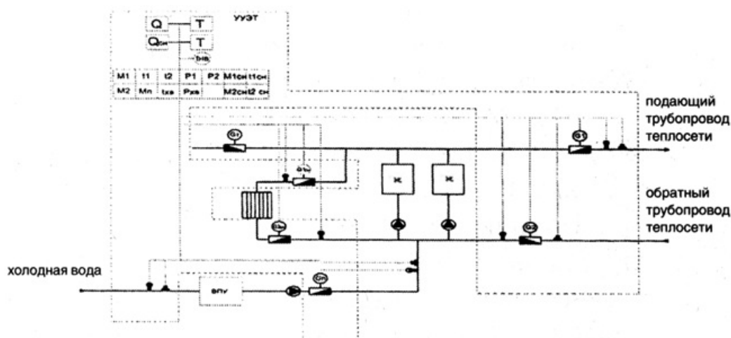
Рисунок 2. Принципиальная схема размещения точек измерения количества тепловой энергии и массы (объема)
